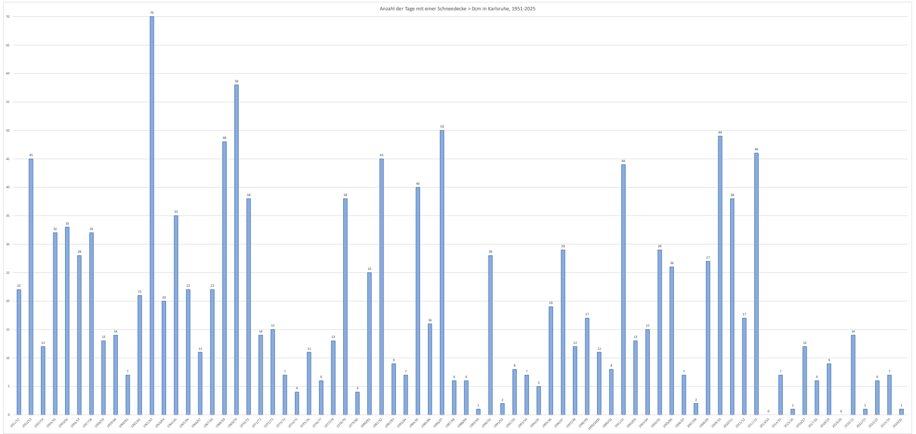
Anzahl der Tage mit einer Schneedecke > 0cm in Karlsruhe, 1951-2025
